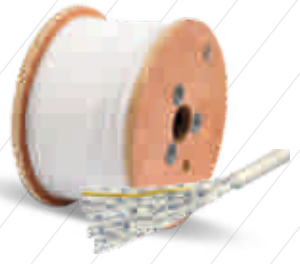
Kuyu Dibi Asansör Kumanda ve Revizyon Kablosu ( Circular Flexible Cable ) 6x0,75 - 8x0,75 - 10x0,75 - 12x0,75
